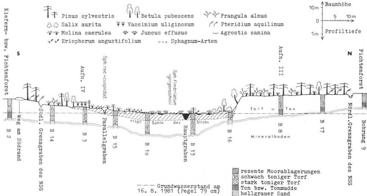
Abb. 6: Querschnitt durch den Westteil des Jägersburger Moors
