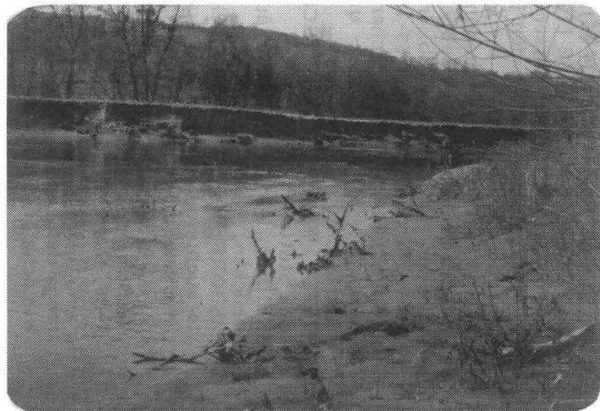
Abb. 13: In Flutmulden der Auewiesen bei Bliesransbach sammelt sich Qualmwasser.
