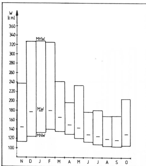
Abb. 2: Wasserstandsschwankungen am Pegel Reinheim zwischen MNW und MHW für den Zeitraum 1959-82
