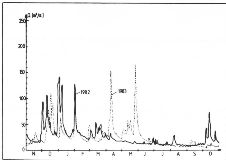
Abb. 3: Abflußganglinien für die Jahre 1982 und 1983 am Pegel Reinheim
