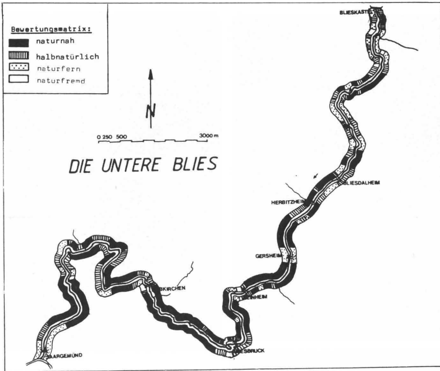
Abb. 8: Gehölzzustand der Blies
